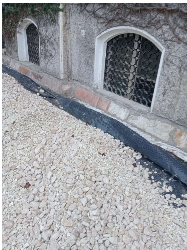
RACCORDO GUAINE CON EDIFICIO
